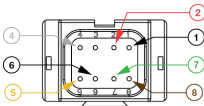
Deutsch DT04-08PA
