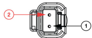
Deutsch DT04-2P
