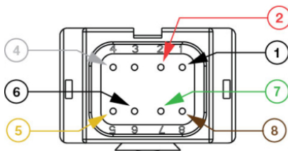
Deutsch DT04-08PA
